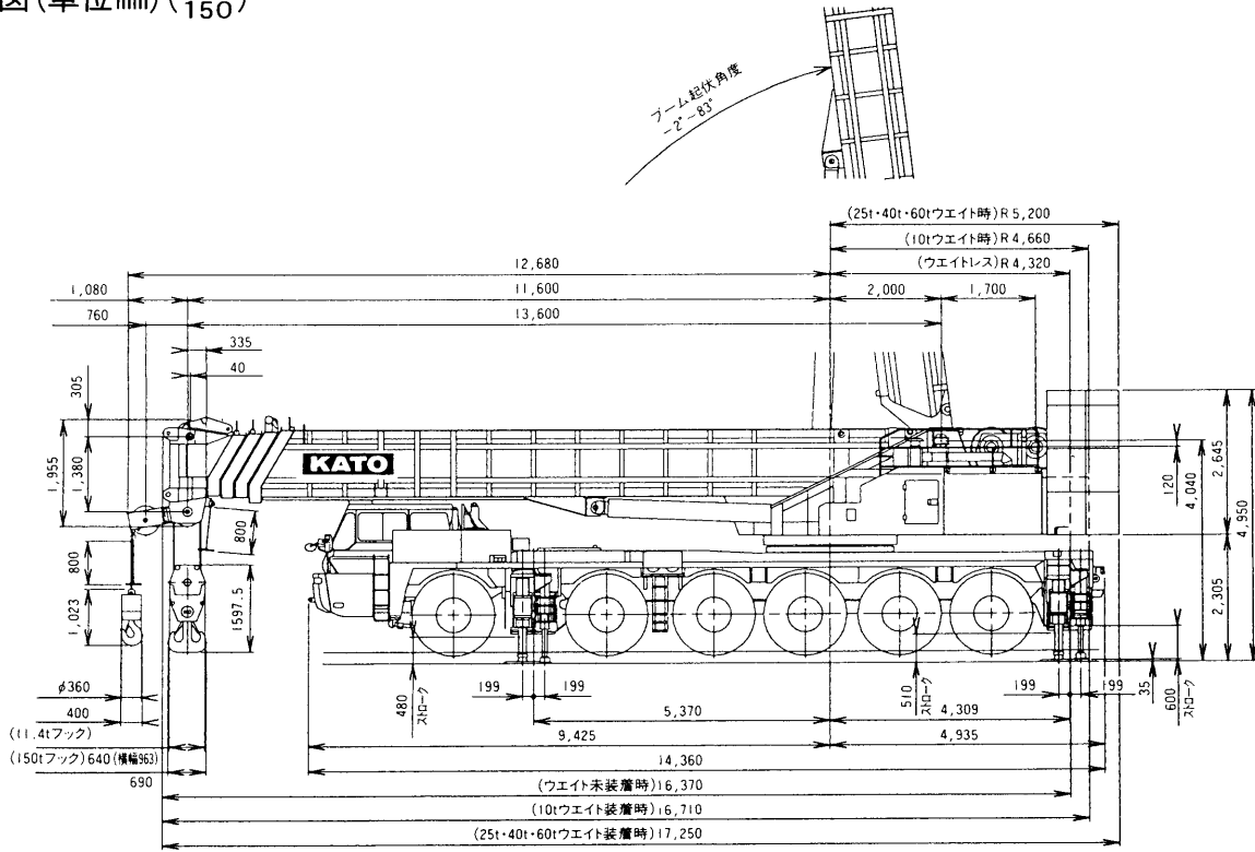
■全体図(単位mm) ( \frac{1}{150} )
